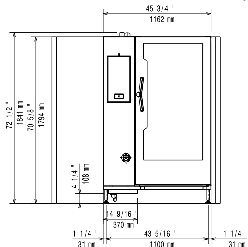
Oldalnézet
